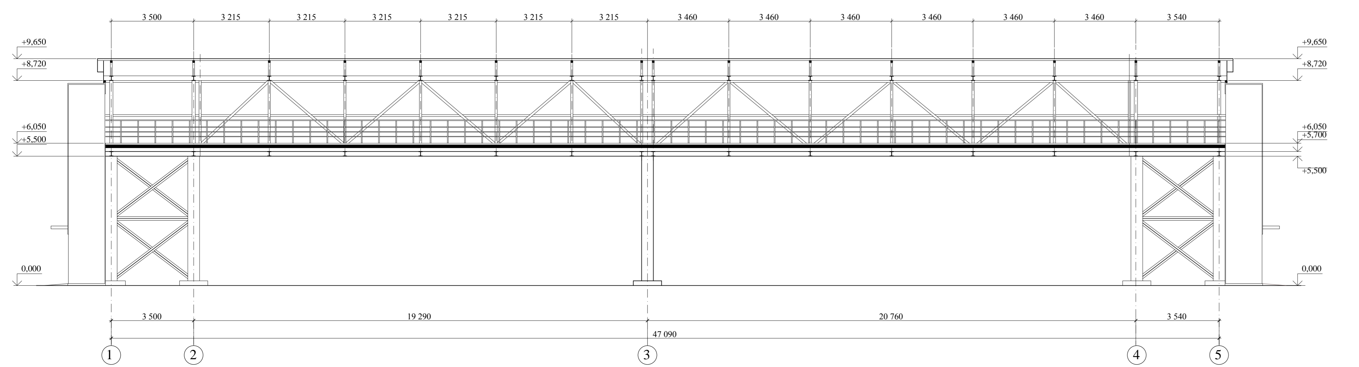
Фасад 1 - 5
