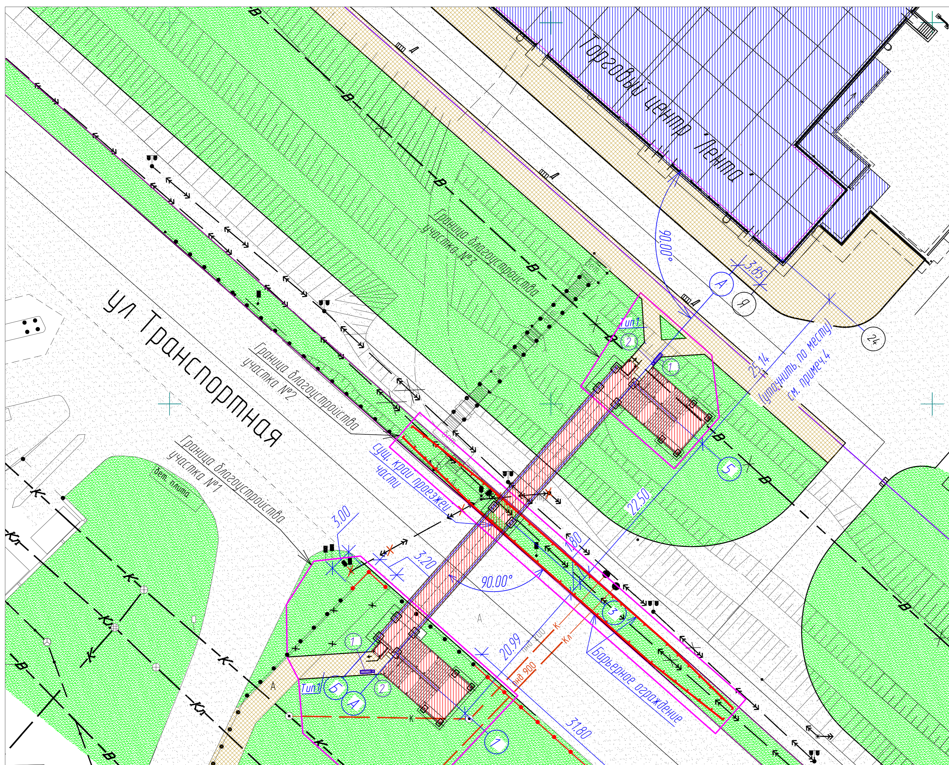
Схема размещения
