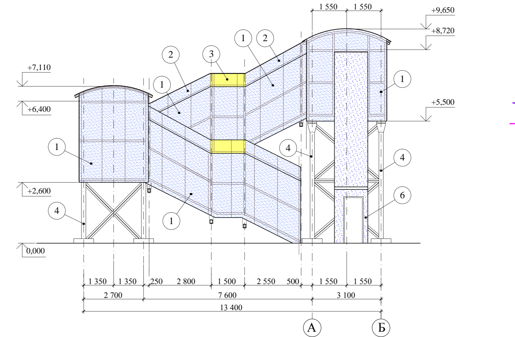
Фасад А - Б
