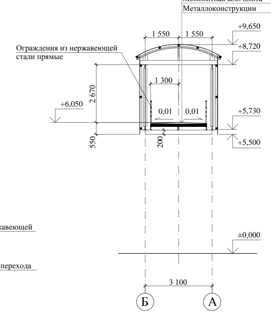
Разрез 3 - 3
