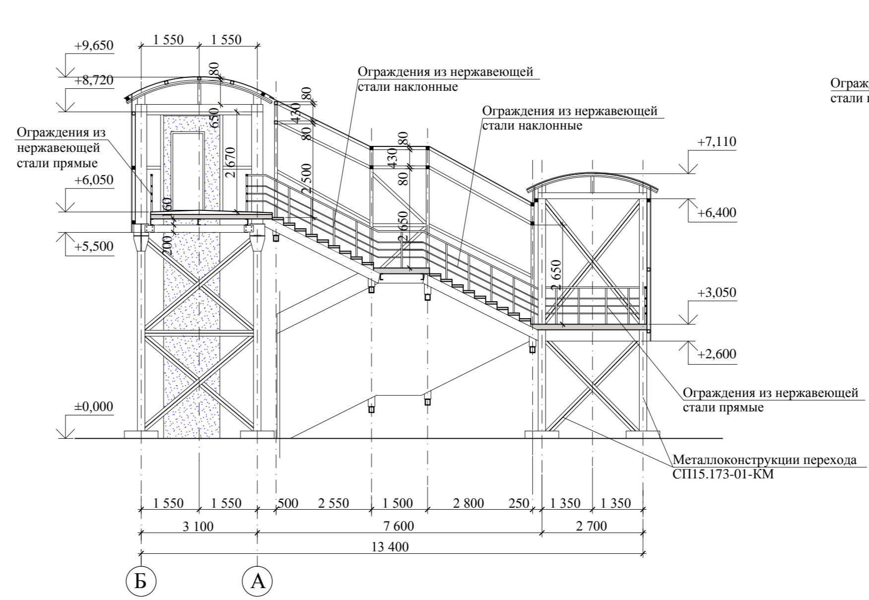
Фасад А - Б
